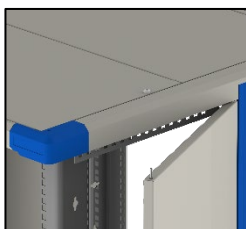
Seitenwand (Verschluss)
